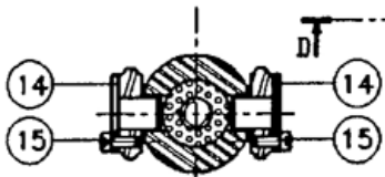
COUPE PARTIELLE C-C REP 13 RAMENE DANS LE PLAN
