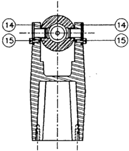
COUPE PARTIELLE B-B REP 13 RAMENE DANS LE PLAN
