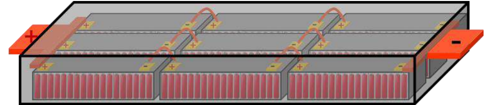
Pack de modules : 3S3P (756 cellules) 68,4 V – 132 Ah – 9 kWh ~ 75 kg
